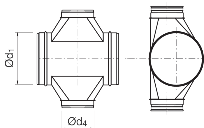
X-KOS X - ekscentričen
