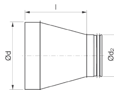
RCFLU - sestavljena izvedba
