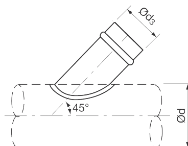
SEDLASTI NASTAVEK PSV
