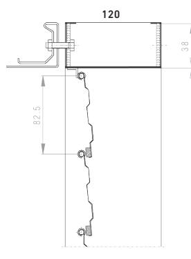
Direktna montaža na kanal (prirobnica)
