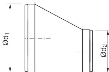
REDUKCIJA DOLGA RL - ekscentrična
