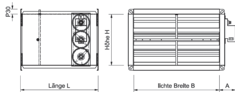
PVSR-EJ - ohne Dämmschale
