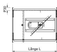
PVSRE-EE - ohne Dämmschale
