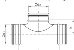
TCPU - centrični prešana izvedba
