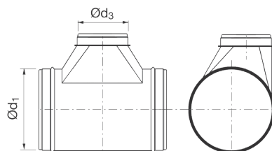
ODCEP T - ekscentričen
