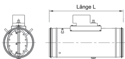
PVSR-R - brez izolacije
