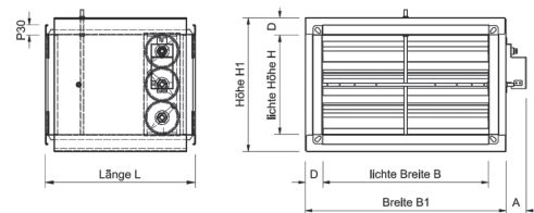
PVSR-EJ/D - mit Dämmschale
