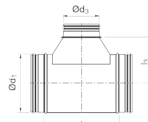
TCU - centrični prešani oz. sestavljeni s prešanim sedlastim nastavkom
