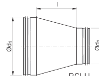
RCLU - sestavljena izvedba
