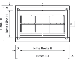
PVSRE-EE/D - mit Dämmschale
