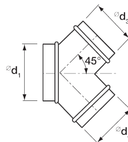
HLAČNI KOS YV
